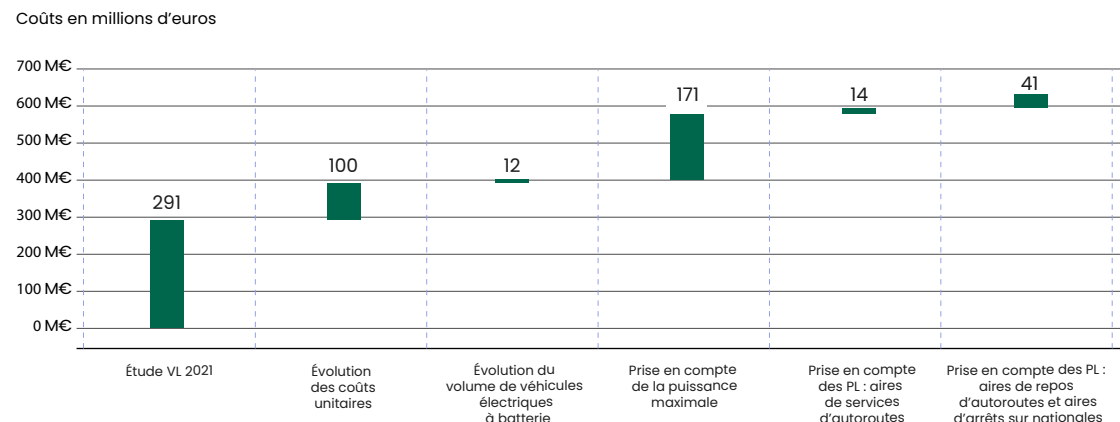
Figure 20 : Évolution des dépenses d'investissement sur le réseau électrique par rapport au scénario de référence de l'étude Enedis/RTE de 2021
