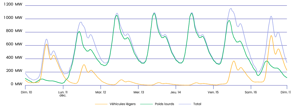
Figure 15 : Courbes hebdomadaires de la puissance de recharge en itinérance d'ici à 2035 pour les VL et les PL (scénario PL BEV haut) lors du pic de recharge des PL
